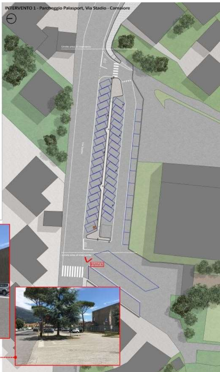
FOTO 1: Veduta d'insieme dell'area prima e dopo l'intervento di progetto
