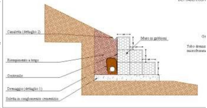
MURI IN GABBIONI SEZIONI TIPO scala 1:100
